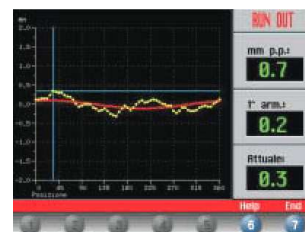
sonar pomiaru niecentryczności
